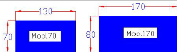
Le Forme RETTANGOLARI Del Piano Stiro Della Serie TRA8-TRA9-FGA8-FGA9 dimensioni in cm
